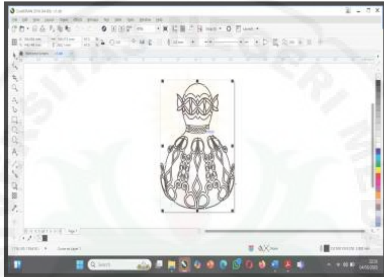
Merancang Desain
