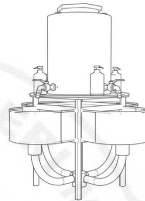
Gambar 7. Ilustrasi 3 Dimensi ‘Wastafel Bundar’.
