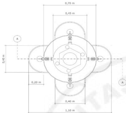
Gambar 4. Denah atau Penampang Atas.
