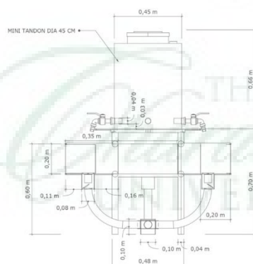
Gambar 6. Potongan ‘Wastafel Bundar’.
