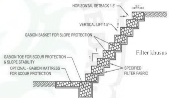
Gambar 21. Gambar Kerja Pemasangan Bronjong (Kementerian Pekerjaan Umum, 2012).
