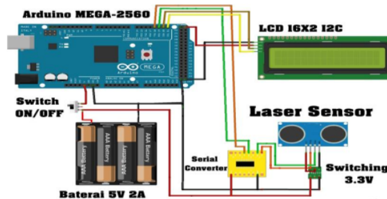
Gambar 2. Rancangan dan Pembuatan Skematik Wiring Sistem
