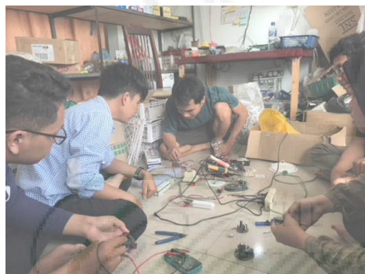
Gambar 6. Proses uji coba akhir setelah perbaikan
