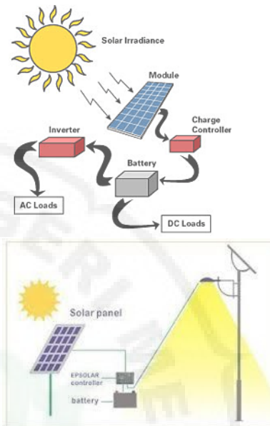
Gambar 5. Skema Lampu Penerangan Tenaga Surya (Siregar et al., 2021) (Surakarta et al., 2019)
