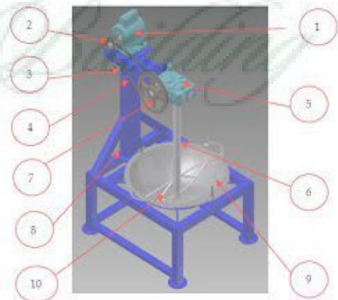
Gambar 3. Desain Alat Pengaduk Dodol Otomatis (Syinnaqof & Riandadari, 2017).
