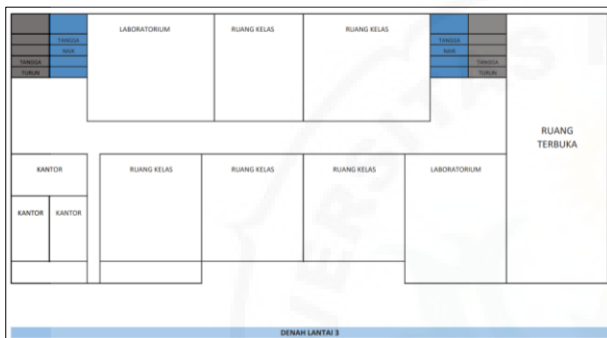
Gambar 3. Denah ruangan lantai 3 SMAS Primbana
