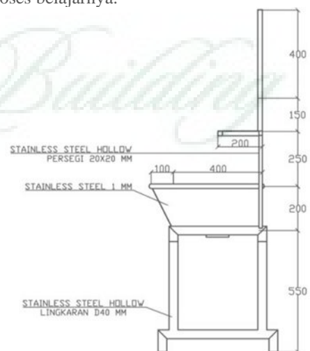
Gambar 9. Hasil desain, bentuk dan model wastafel
