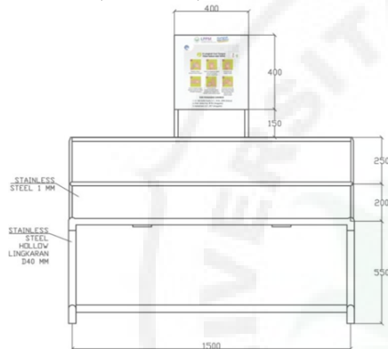
Gambar 5. Tampak Depan Wastafel, skala 1:20
