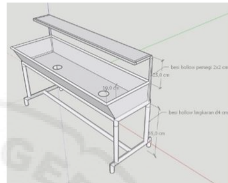
Gambar 8. Spesifikasi bentuk dan bahan
