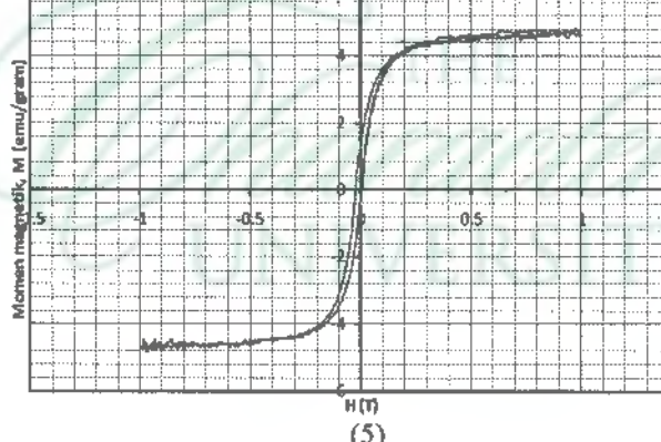
Gambar 2. Kurva Histeresis Nanopartikel Fe_3O_4 (2), nanokomposit Fe_3O_4 -Montmorilonit pada suhu 40^\circ C (3), 70^\circ C (4), 100^\circ C (5)
