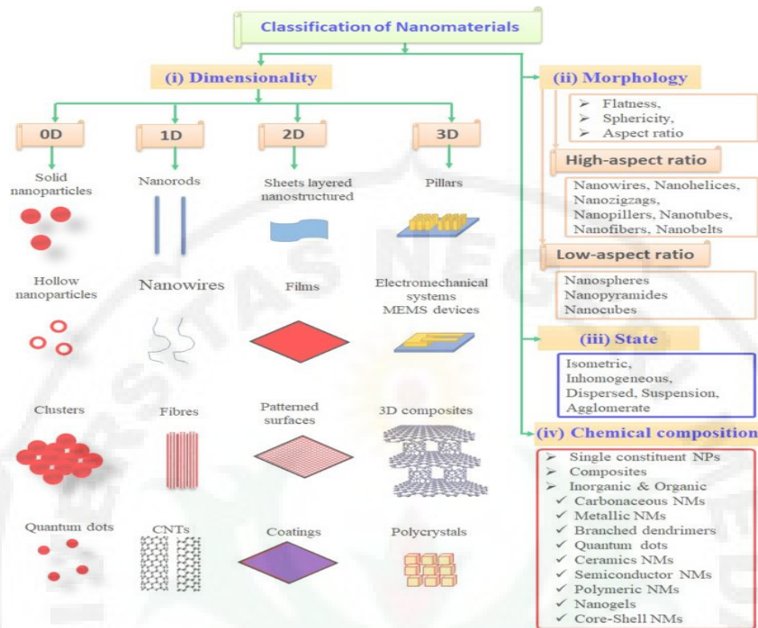
Gambar 2. Klasifikasi nanomaterial [6].
