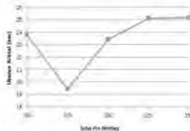
Gambar 2. Pengaruh Kenaikan Suhu Pre-heating terhadap Ukuran Kristal
