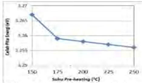
Gambar 2. Grafik Pengaruh Suhu Pre-heating terhadap Celah Pita Energi
