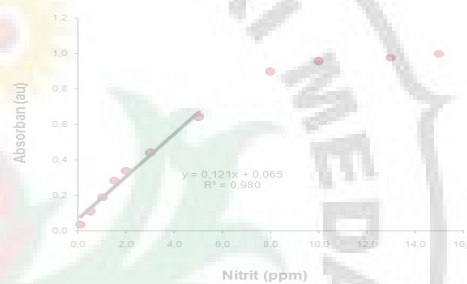
Gambar 6. Kurva kalibrasi larutan standar 1-15 mM nitrit diukur pada \lambda 542 nm di dalam larutan buffer posfat 0,01 M pada pH 3,0.
