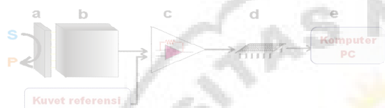
Gambar 4. Rancang bangun sensor kimia dalam sistem statis yang terdiri atas: analit (nitrit): (a) senyawa kimia aktif (sulfanilat) terimobilisasi didalam polityramin, (b) transduser pewarna N-(1-naftil) etilen diamin dihidroklorida (NED), (c) Kuvet terintegrasi di dalam double beam spektrofotometry UV-Vis, (d) amplifikasi signal, dan (e) signal prosessor pada komputer PC. Dalam analisis ini S = substrat, dan P = Produk
