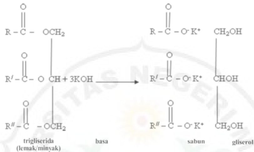
Gambar 3. Persamaan reaksi penyabunan
