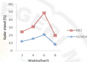
Gambar 5. Grafik hubungan antara waktu fermentasi vs kadar etanol (%)
