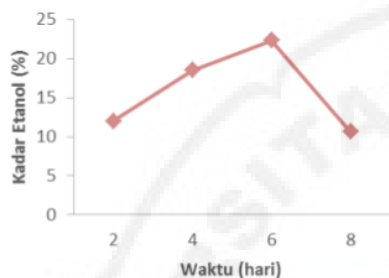
Gambar 3. Grafik hubungan antara waktu fermentasi VS kadar etanol (%).
