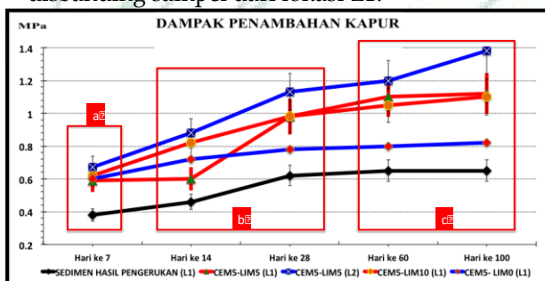
Gambar 2. Percobaan daya Tekan
