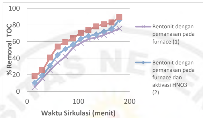
Gambar 2. Pengaruh Waktu Sirkulasi Terhadap Penyisihan TOC
