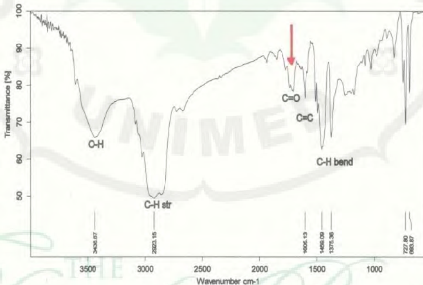
Gambar 2. Spektra FTIR karet alam siklo grafting MA (CNR-g-MA)
