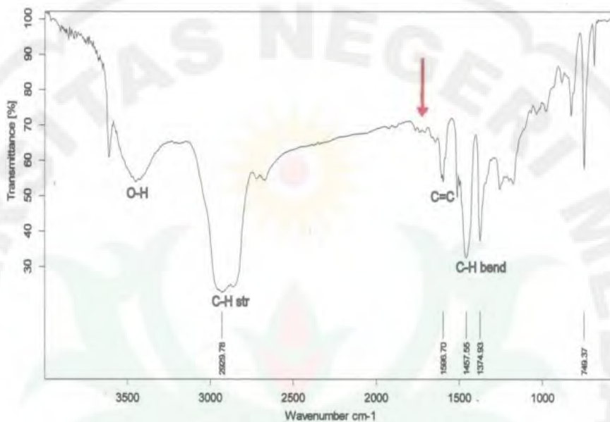
Gambar 1. Spektra FTIR karet alam siklo (resipren-35)
