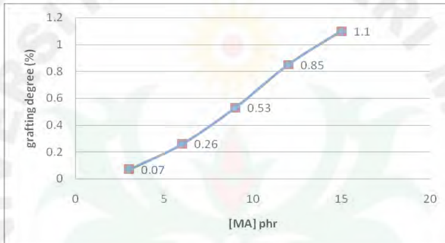
Gambar 3 Konsentrasi MA versus derajat grafting
