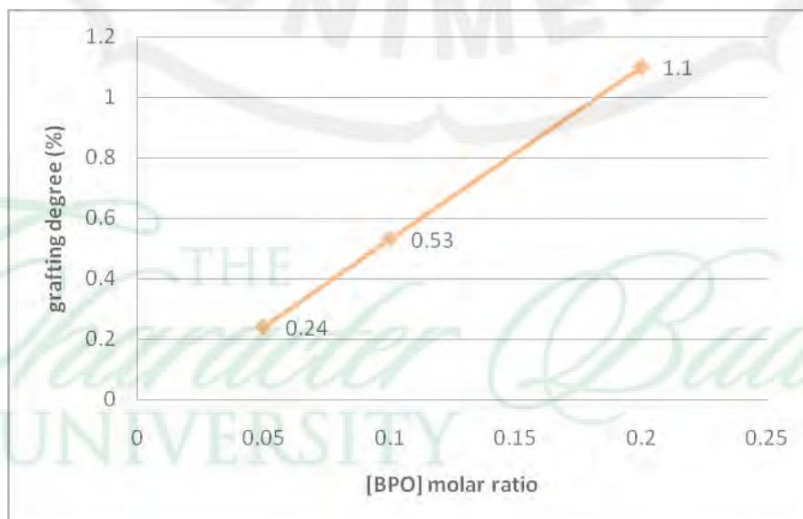
Gambar 4 Grafik Konsentrasi BPO vs derajat grafting
