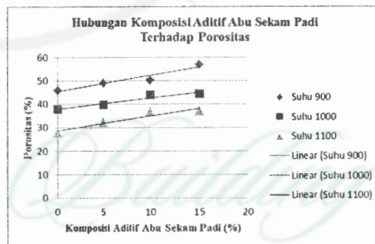
Gambar 3. Hubungan Komposisi Aditif Abu Sekam Padi vs Porositas
