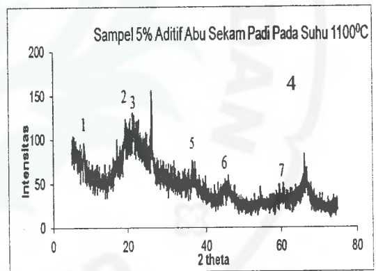
Gambar 6. Pola XRD 5% aditif abu sekam padi pada suhu sintering 1100°C.
