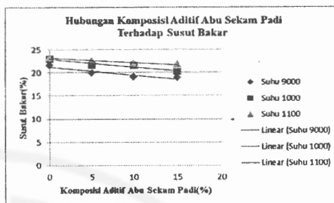
Gambar 1. Hubungan Komposisi Aditif Abu Sekam Padi vs Susut Bakar
