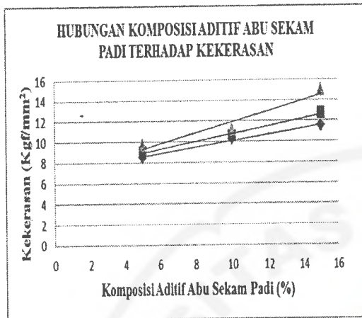
Gambar 5. Hubungan Komposisi Aditif Abu Sekam Padi vs Kekerasan
