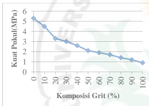
Gambar 8. Grafik hubungan antara kuat pukul terhadap komposisi grit menggunakan PVA
