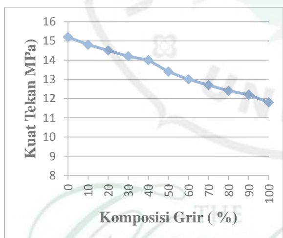
Gambar 6. Grafik hubungan antara kuat tekan terhadap komposisi grit menggunakan PVA. Dari gambar 5 dan 6 (dari kedua grafik) dapat diambil kesimpulan bahwa dengan penambahan grit pada komposisi dari 0% sampai 100% (volume) dan pengurangan pasir dari komposisi dari 100% sampai 0% (volume), penyerapan air semakin besar
