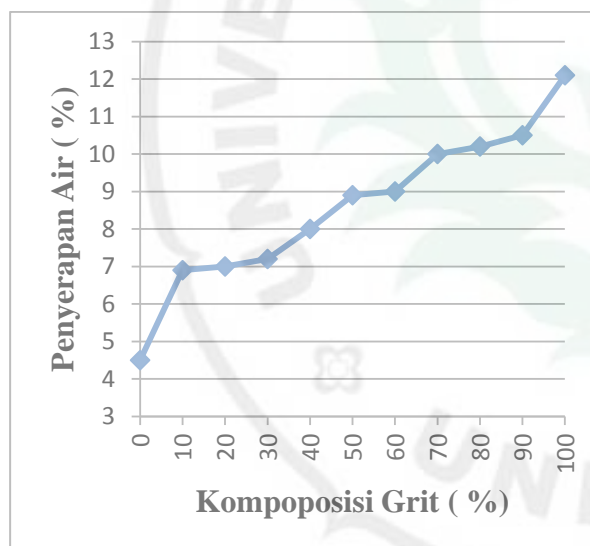
Gambar 3..Grafik hubungan antara penyerapan air terhadap komposisi grit tanpa menggunakan PVA
