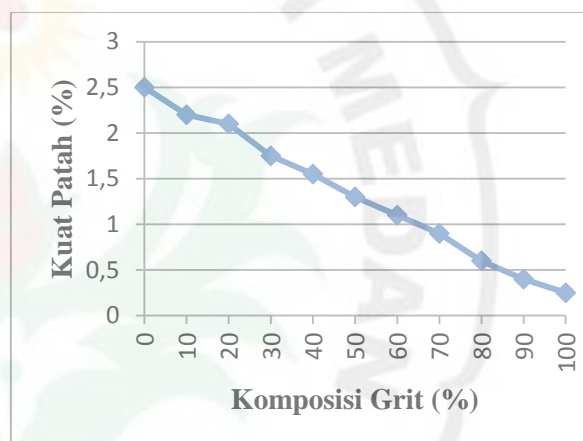
Gambar 9. Grafik hubungan antara kuat patah terhadap komposisi grit tanpa menggunakan PVA
