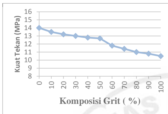
Gambar 5 Grafik hubungan antara kuat tekan terhadap komposisi grit tanpa menggunakan PVA. Hasil pengukuran kuat tekan paving block yang berbasis semen, pasir, grit , PVA ditunjukkan pada gambar 6 dengan variasi komposisi: 0 – 100 % (volume) grit , terlihat diperoleh berkisar antara 15,20MPa – 11,80 Mpa
