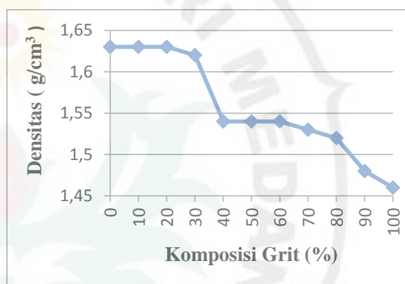
Gambar 2. Grafik hubungan antara Densitas terhadap komposisi Grit dengan menggunakan PVA
