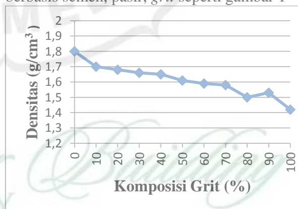
Gambar 1. Grafik hubungan antara Densitas terhadap komposisi Grit tanpa PVA
