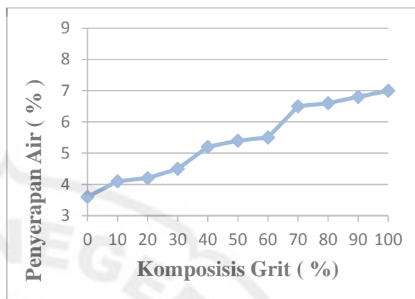
Gambar 4. Grafik hubungan antara penyerapan air terhadap komposisi grit menggunakan PVA
