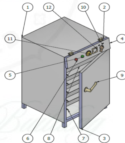
Gambar 3. Alat Pengering Bunga Telang.
