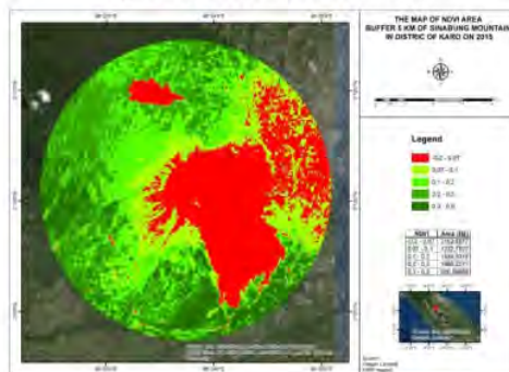
Figure 2.b NDVI Landsat 8 Oli in 2015
