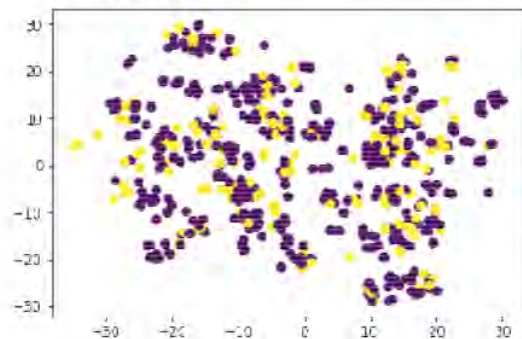
Fig. 5. t-SNE map
