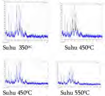
Gambar 2. Analisis XRD
