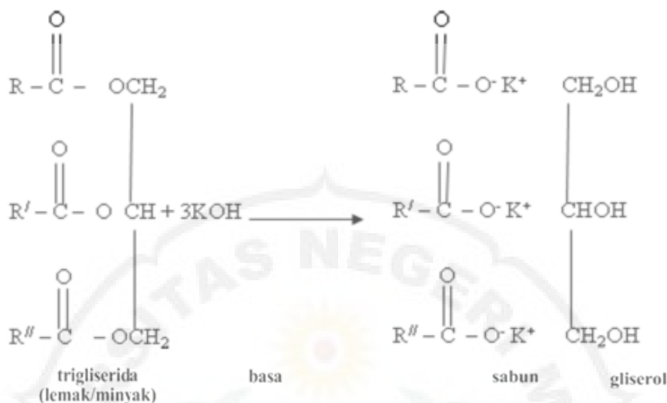
Gambar 3. Persamaan reaksi penyabunan
