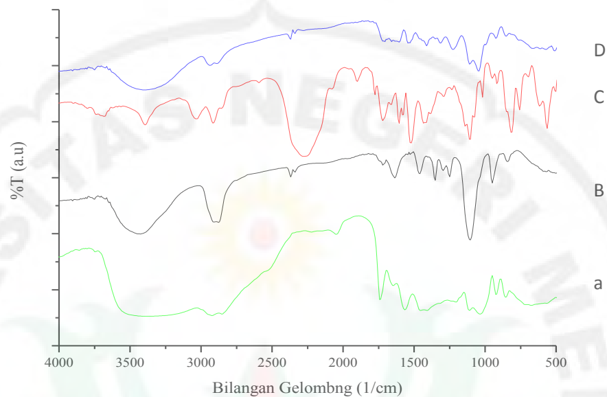
Gambar 2. Spektra IR Pembentukan poliuretan, a. Gliserol, b. PEG 1000, c. MDI, dan d. Poliuretan
