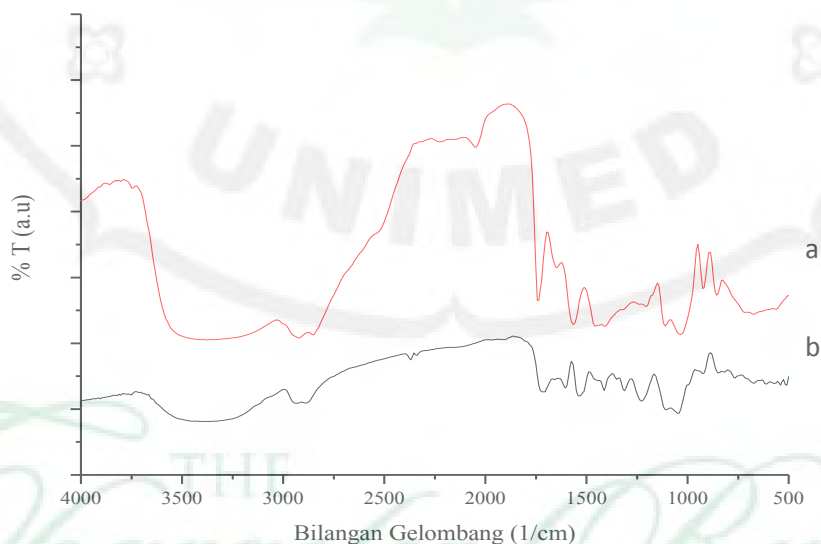
Gambar 1. Spektra IR dari a. Gliserol murni, b. Gliserol dari minyak jelantah
