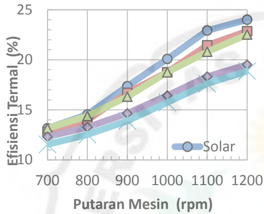
Gambar 4. Efisiensi termal vs putaran mesin
